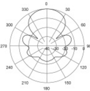
H-Plane | 395 MHz
