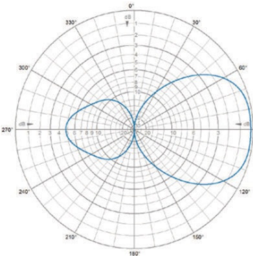
E-Plane | 78 MHz
