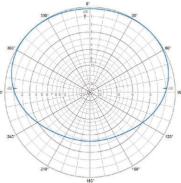
H-Plane | 78 MHz
