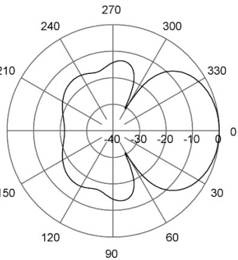
H-Plane | 232 MHz
