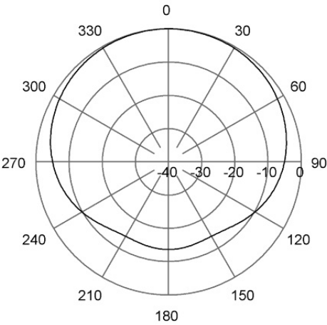
H-Plane | 410 MHz
