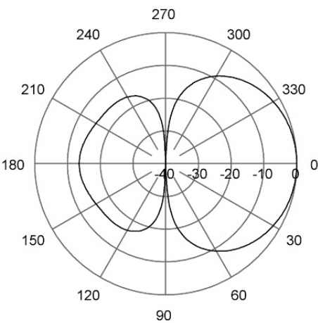
E-Plane | 410 MHz
