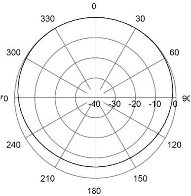
H-Plane | 459 MHz
