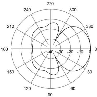
H-Plane | 330 MHz
